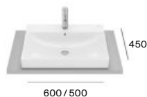
Ona A32768N00J 600x450 A32768L00J 500x450
